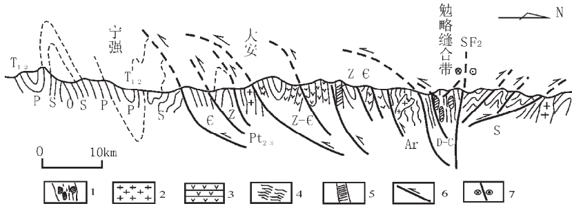
图3 勉略带勉略区段构造剖面图
