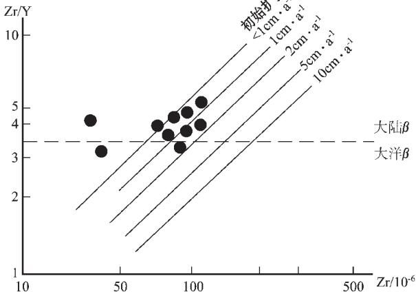
图5 库地蛇绿岩中玄武岩 Zr/Y-Zr 判别图
