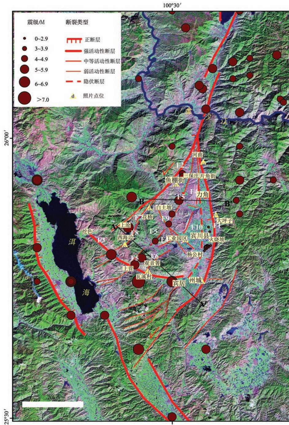
图4 宾川地区断层遥感解译
