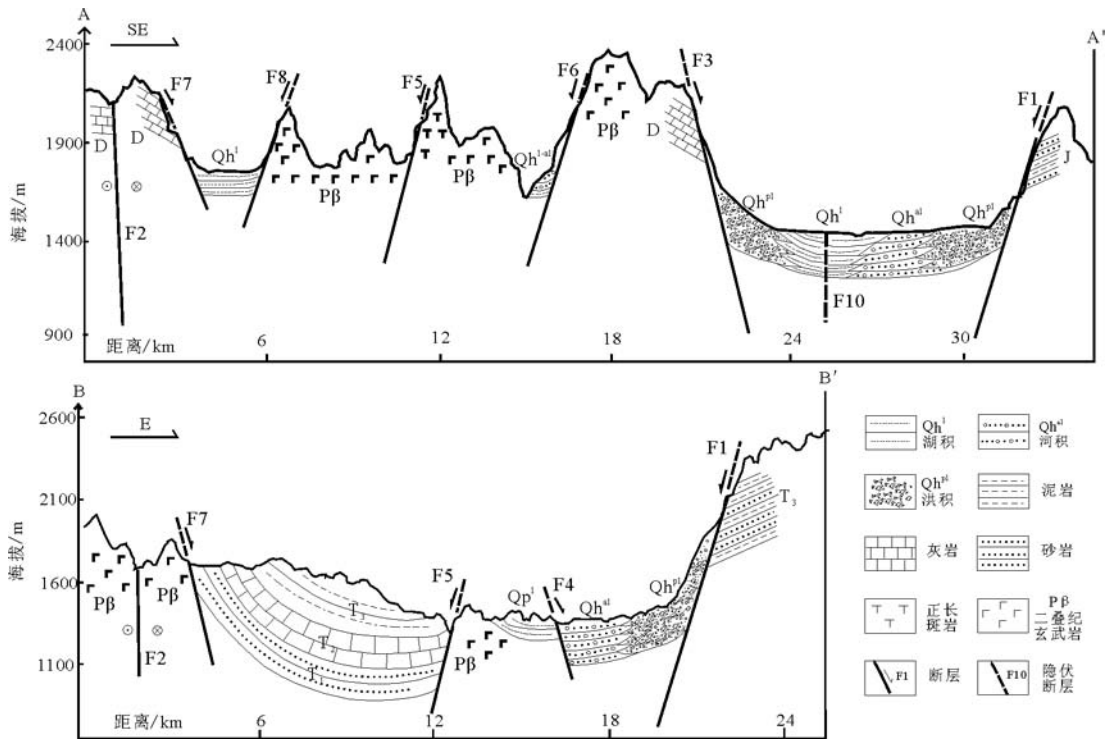
图5 宾川地区A—A'、B—B'地质剖面
