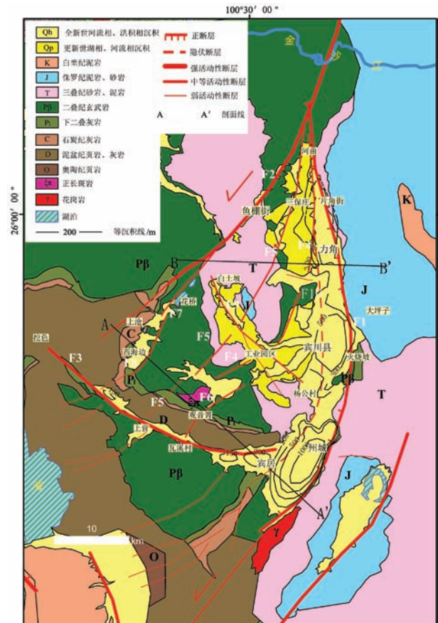
图2 宾川地区地质和第四纪等沉积线图 ① Fig. 2 Geological and Quaternary sedimentary isobath map of Binchuan area
