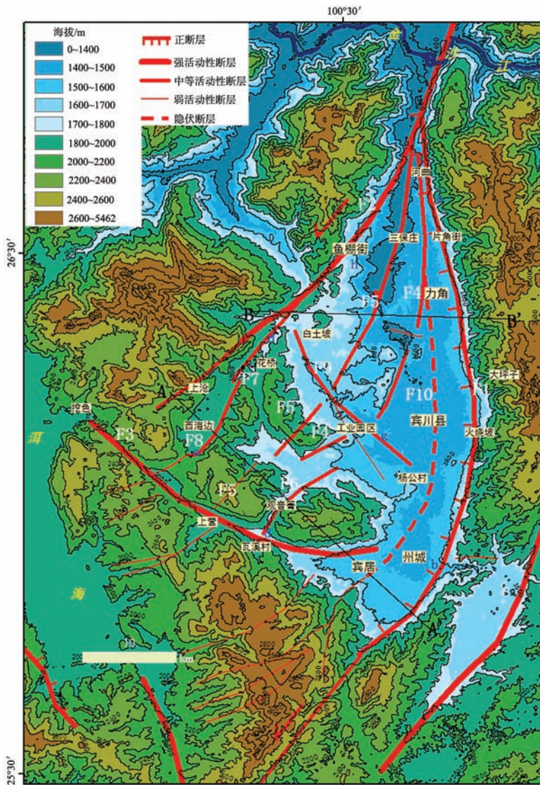
图3 宾川地区地形图
