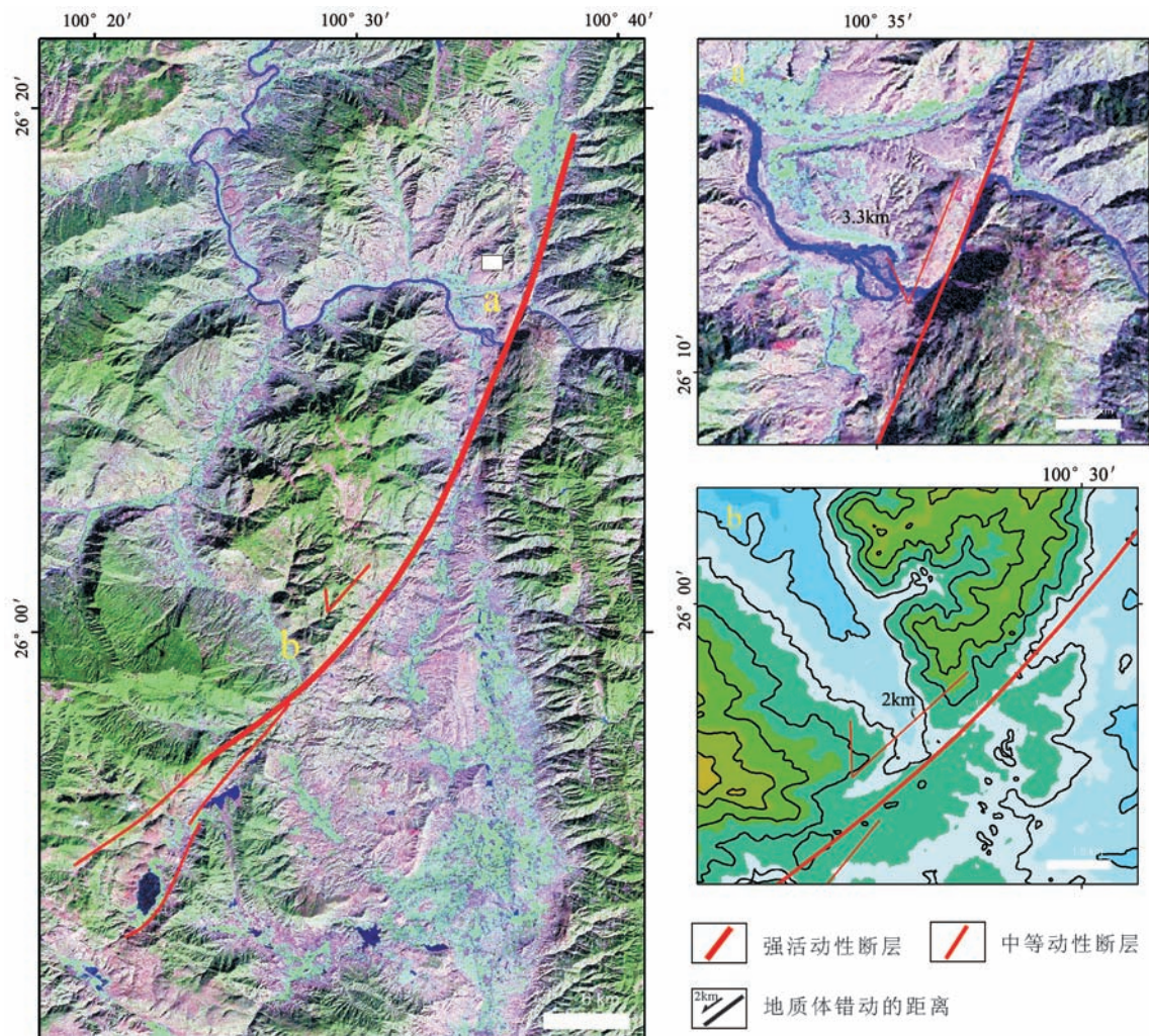
图6 F2左旋错动地质体图示
