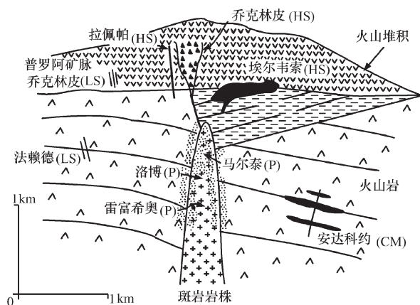
图7 智利若干典型金矿床相对于理想化斑岩系统的产出位置 [14]
