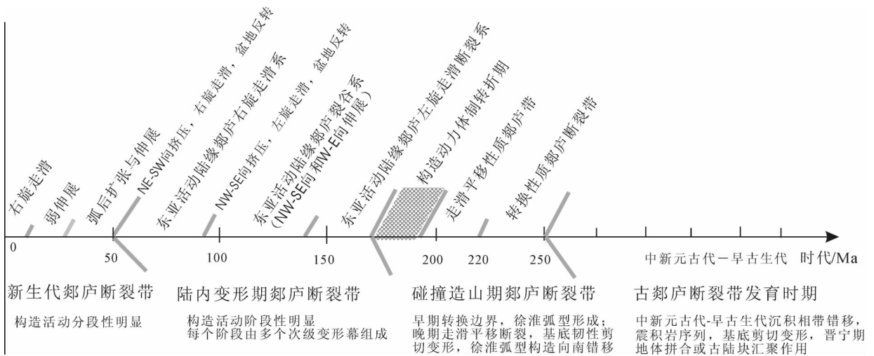
图8 郟庐断裂带构造演化阶段划分示意图
