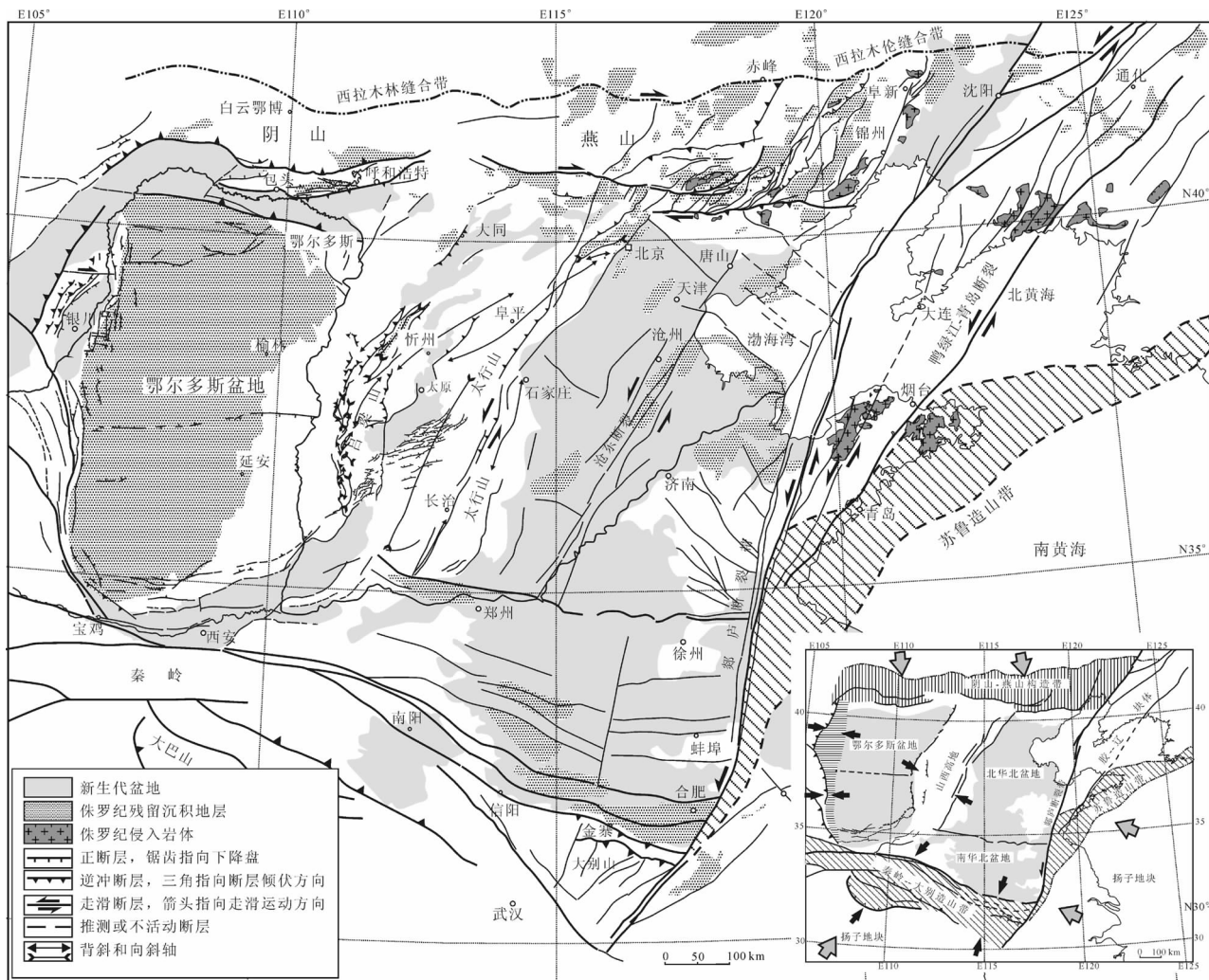
图 7 华北侏罗纪构造纲要图 [80]
