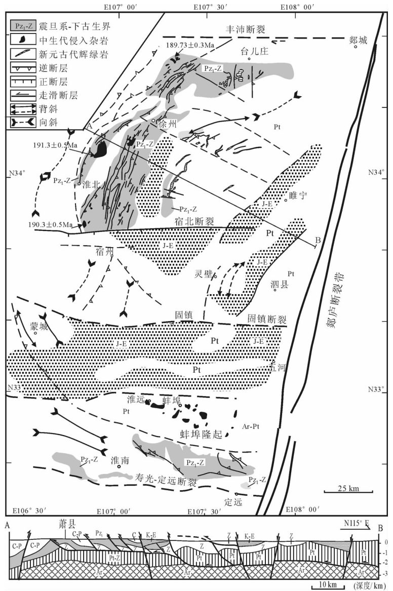
图 4 徐淮弧型构造简图(位置见图 1)
