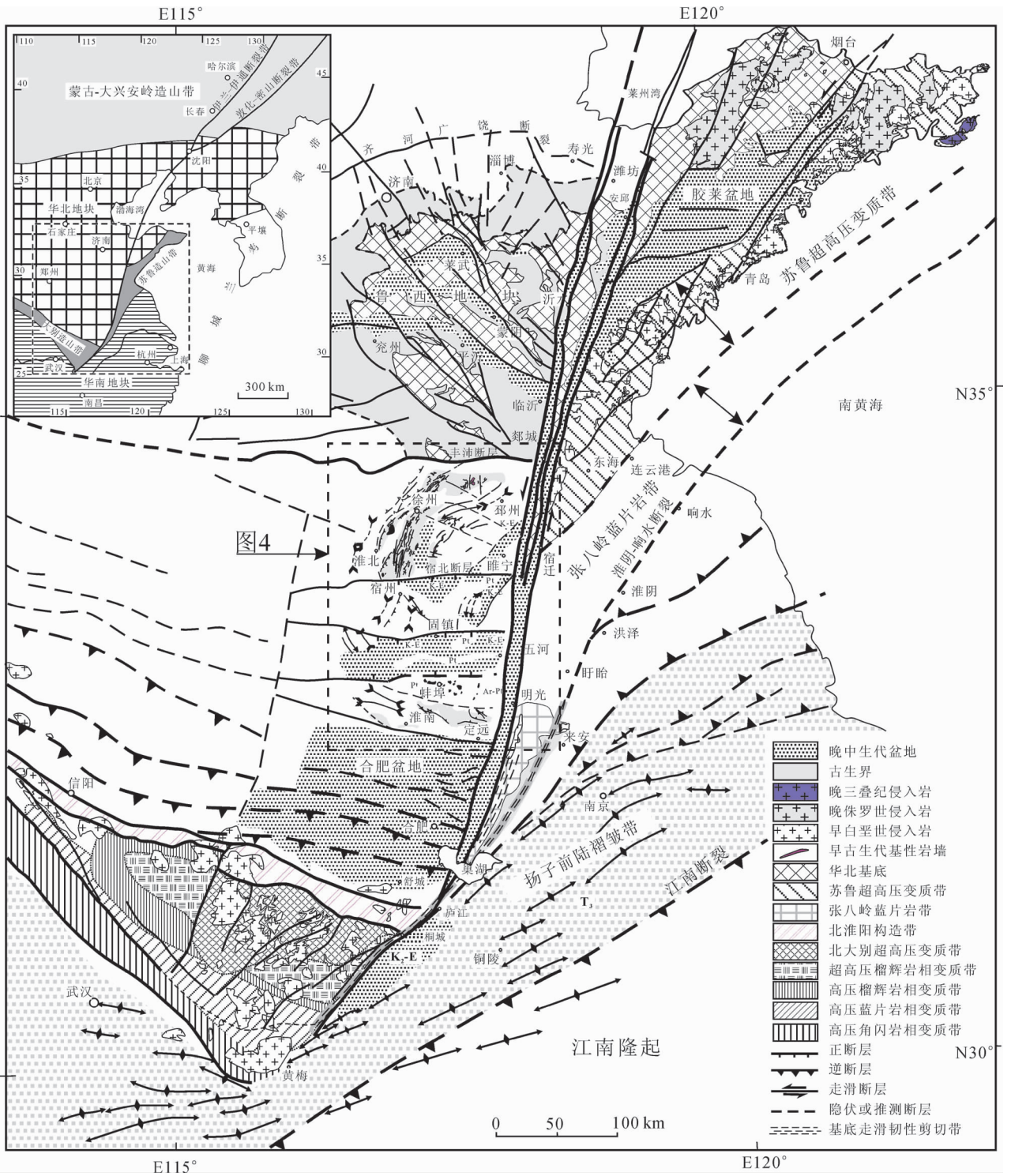
图 1 郯庐断裂带中南段构造纲要图(根据参考文献[39-43]编制)
