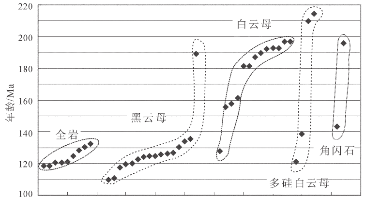
图 2 郟庐断裂带基底韧性走滑剪切带 40 Ar- 39 Ar 测年数据散点图 (据参考文献[8-9,35-36,38-39,48])
