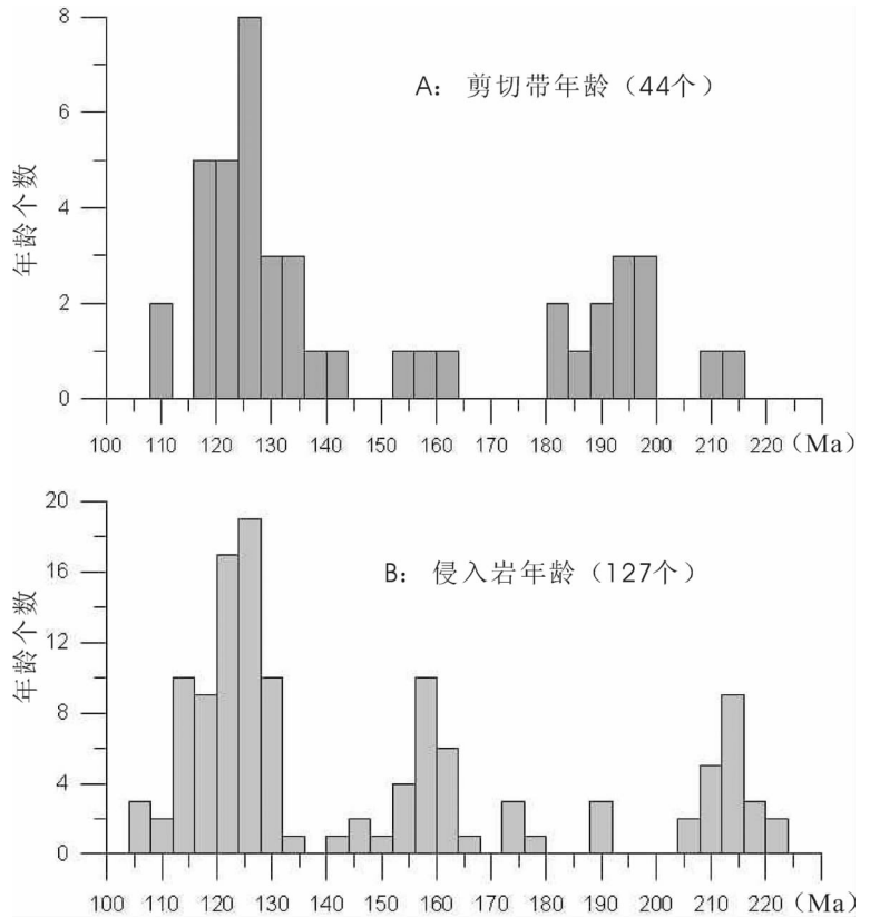
图 3 郟庐断裂带基底韧性剪切带 40 Ar- 39 Ar 测年数据直方图(A) 和断裂带两侧中生代侵入岩体同位素年龄数据直方图 (B) (据参考文献[8-9,35-36,38-39,48])
